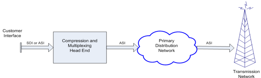
Γράφημα 1: Σχηματικό Διάγραμμα Δικτύου Velister
