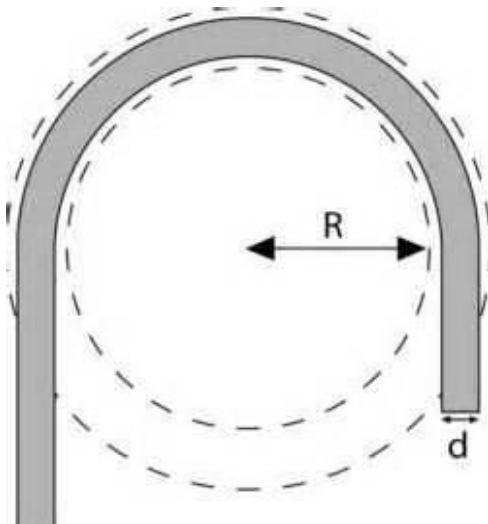
Σχήμα 7 ακτίνα κάμψης
