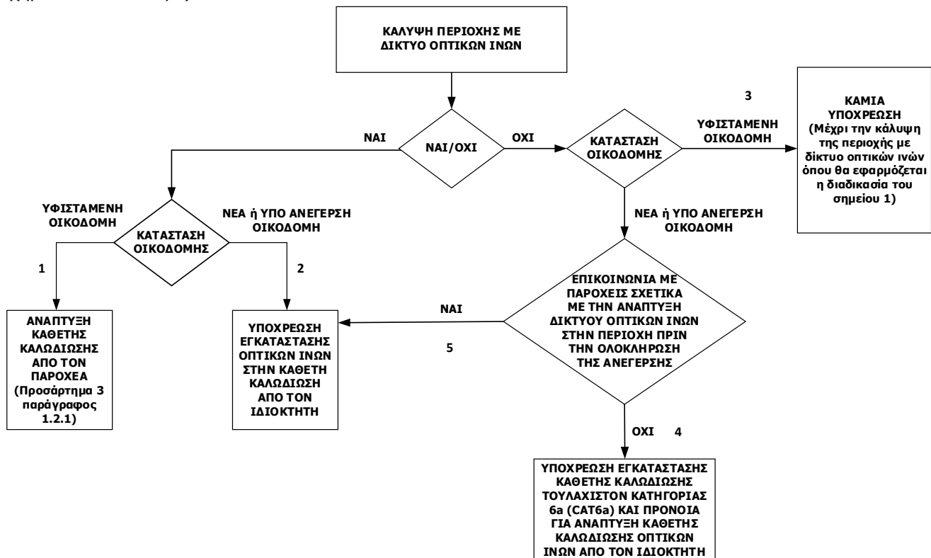
Σχήμα 1. Ανάπτυξη κατακόρυφης καλωδίωσης σε οικοδομές
