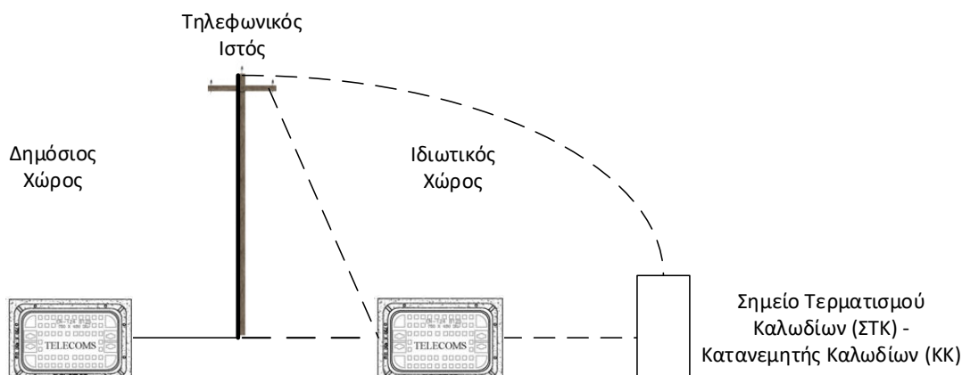
Σχήμα 2: Προσβάσεις προς την οικοδομή από το δημόσιο δίκτυο
