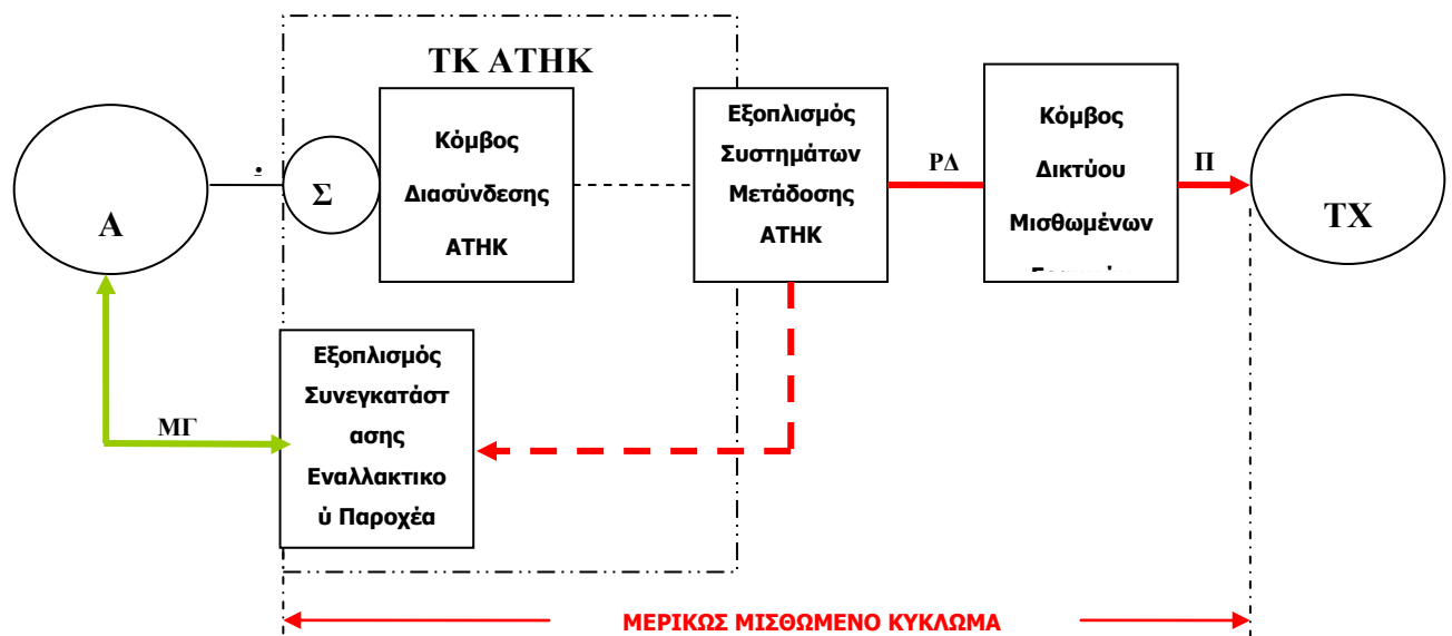
Διάγραμμα 4: Συνδεσμολογία Παροχής Πολλαπλών Μερικώς Μισθωμένων Κυκλωμάτων Ρυθμού Μετάδοσης 2 Mbit/s
