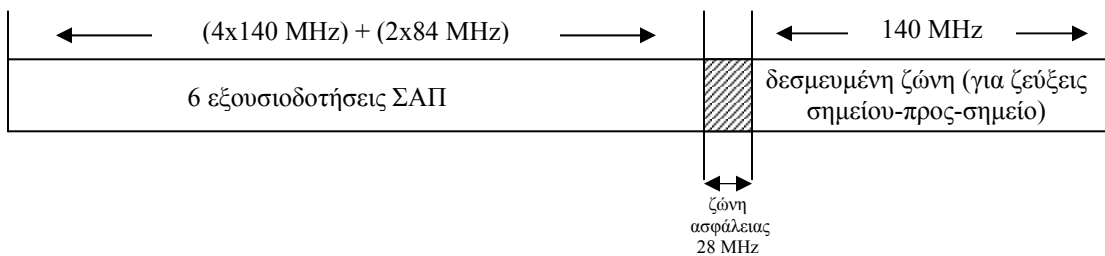
Σχήμα 4: Κατανομή μιας υποζώνης στη ζώνη 24.5 – 26.5 GHz.
